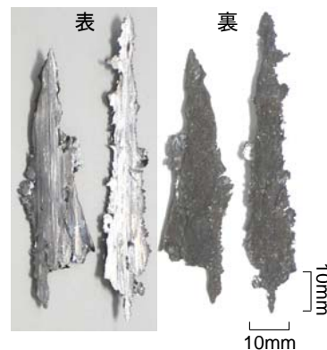
図2 現車のかじり鉄片
