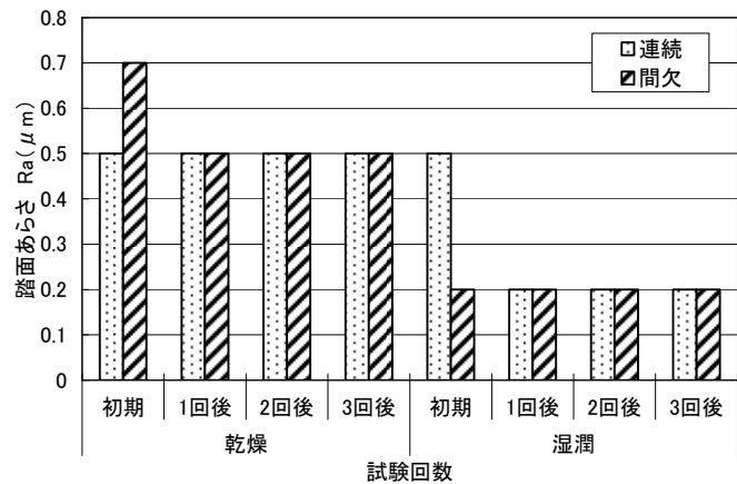
図 8 あらしの測定結果
