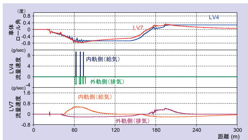
図 急曲線通過中の車体ロール角と高さ調整弁の動作状況 (半径: 160m カント: 95mm 速度: 10km/h)
