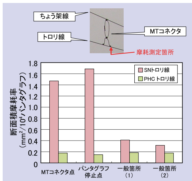
図5 トロリ線の摩耗率(新幹線駅構内)
