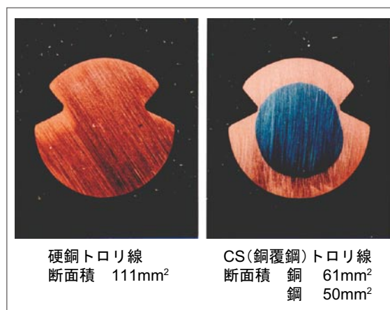
図1 硬銅トロリ線とCS(銅覆銅)トロリ線
