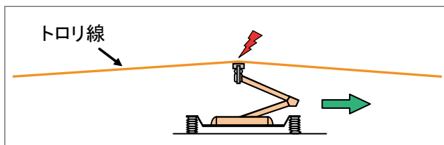
図7 パンタグラフ通過に伴うトロリ線曲げひずみ発生イメージ
