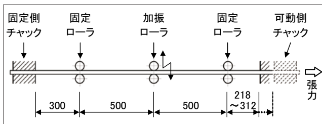
図8 トロリ線疲労試験装置概略
