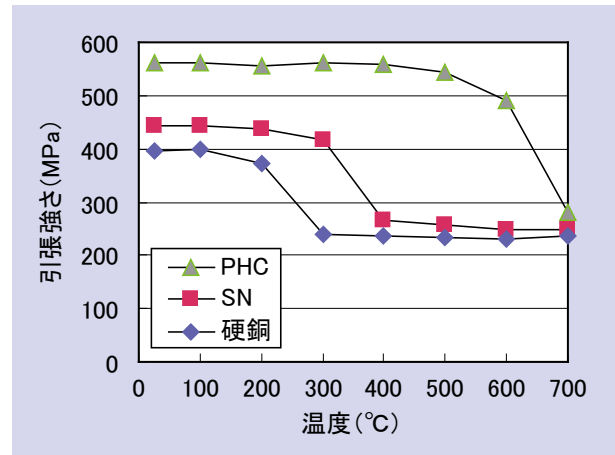
図4 各種トロリ線材料の焼鈍軟化特性
