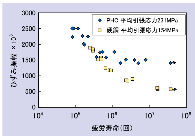
図9 トロリ線疲労試験結果 (→は未破断で試験打ち切り)
