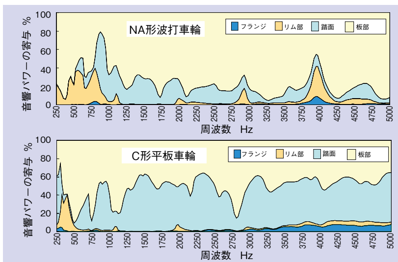
図 構造音場解析による車輪の音響パワー寄与
