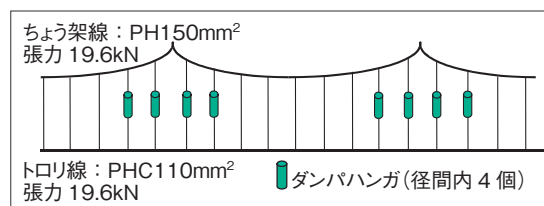
図1 PHCシンプル架線の構造
