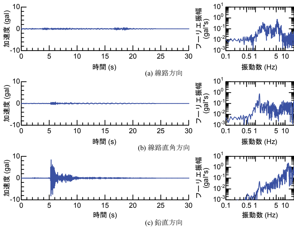
付図4-130 地震観測記録（地震No. 27, R4S-1観測点）
