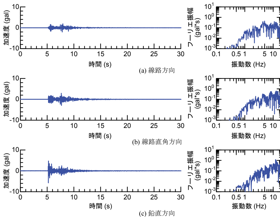
付図4-133 地震観測記録（地震No. 28, R4G観測点）
