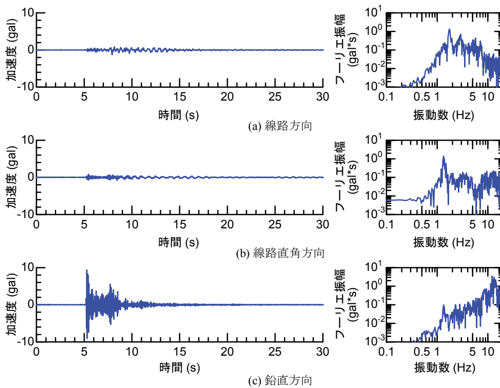
付図4-134 地震観測記録（地震No. 28, R4S-1観測点）
