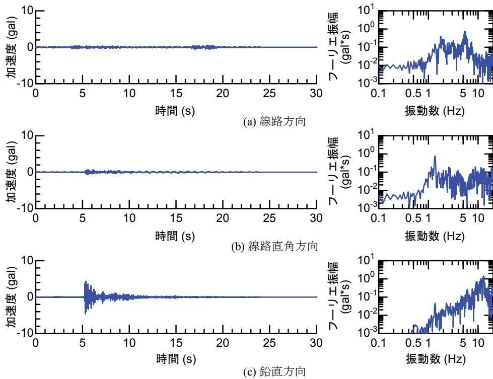
付図4-131 地震観測記録（地震No. 27, R4S-2観測点）
