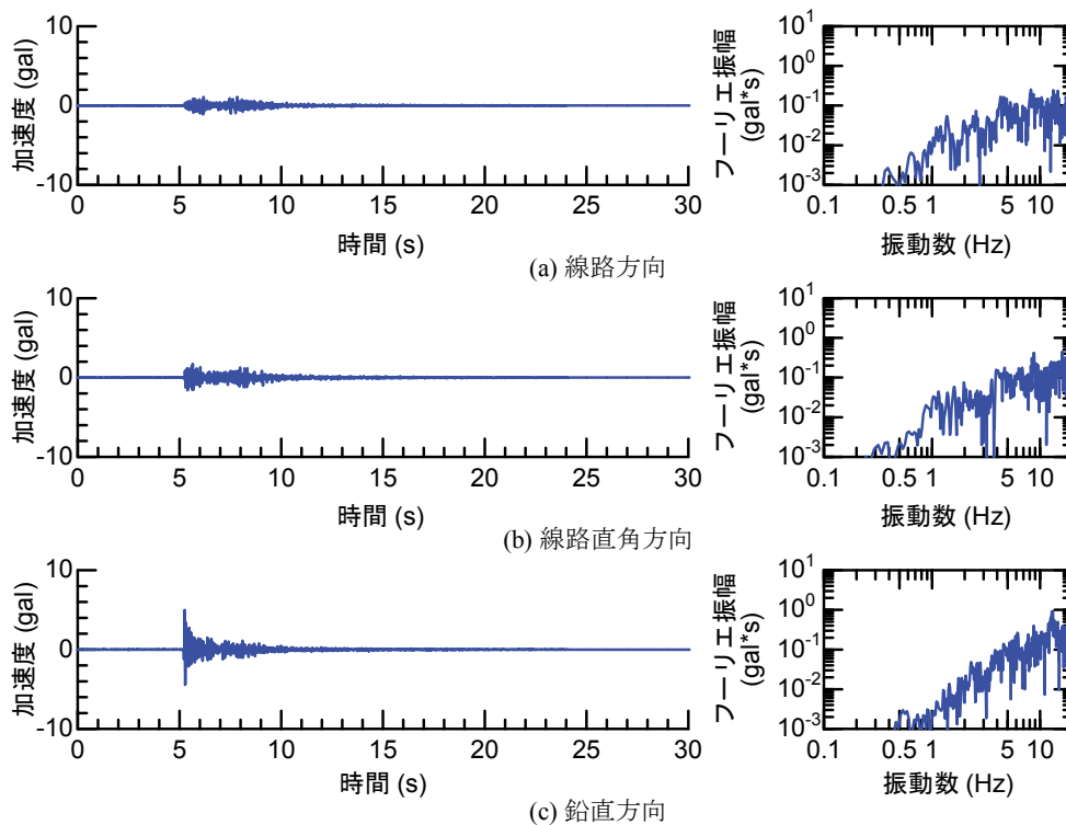
付図4-128 地震観測記録（地震No. 27, R4G観測点）
