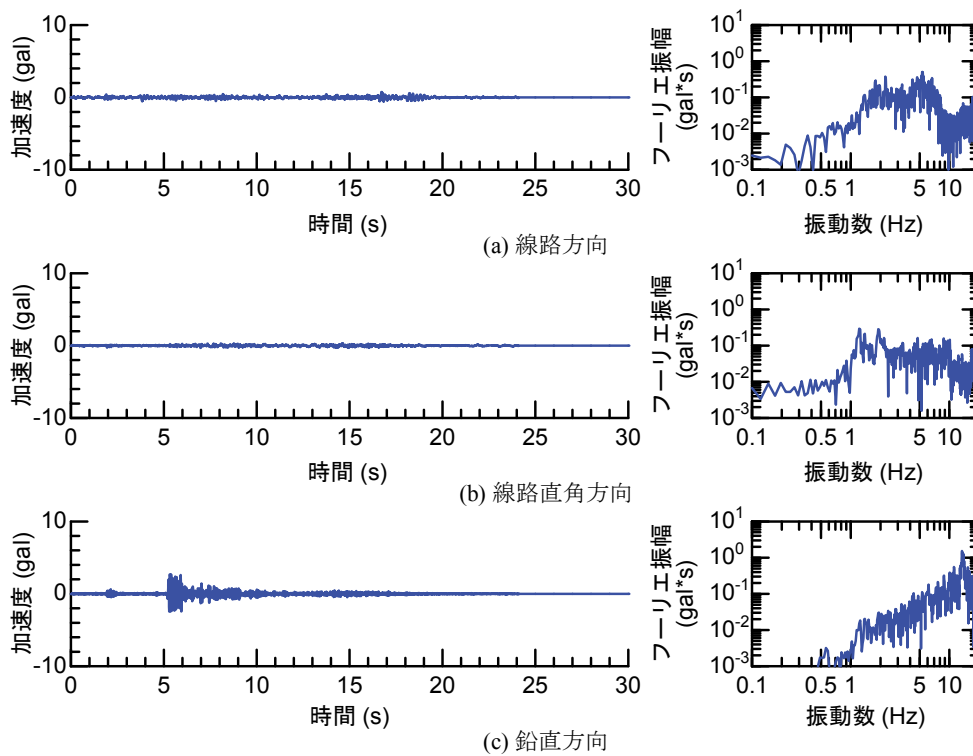
付図4-129 地震観測記録（地震No. 27, R1S観測点）
