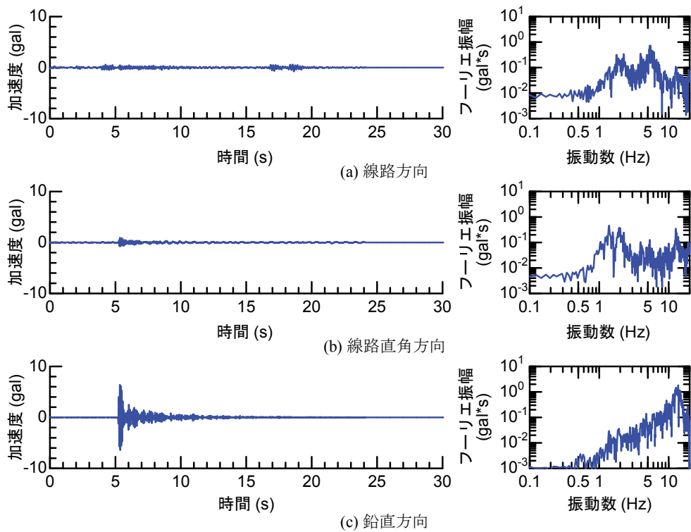
付図4-132 地震観測記録（地震No. 27, R6S観測点）
