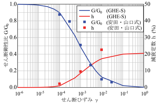
(g) No. 9層
