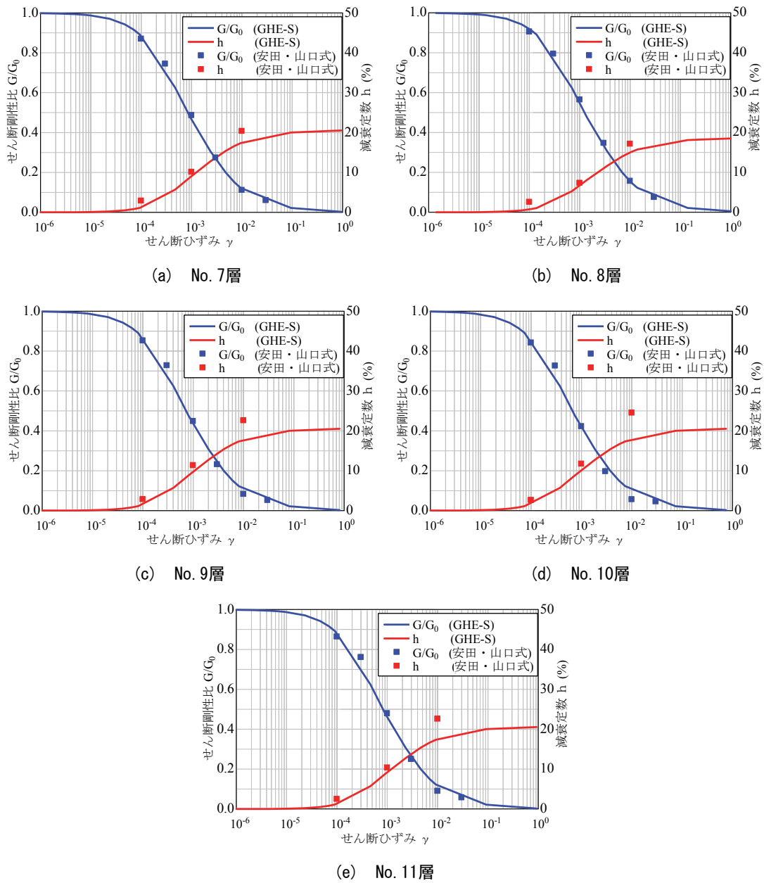
付図2-2 動的変形特性の設定結果（在来線地震計）その2
