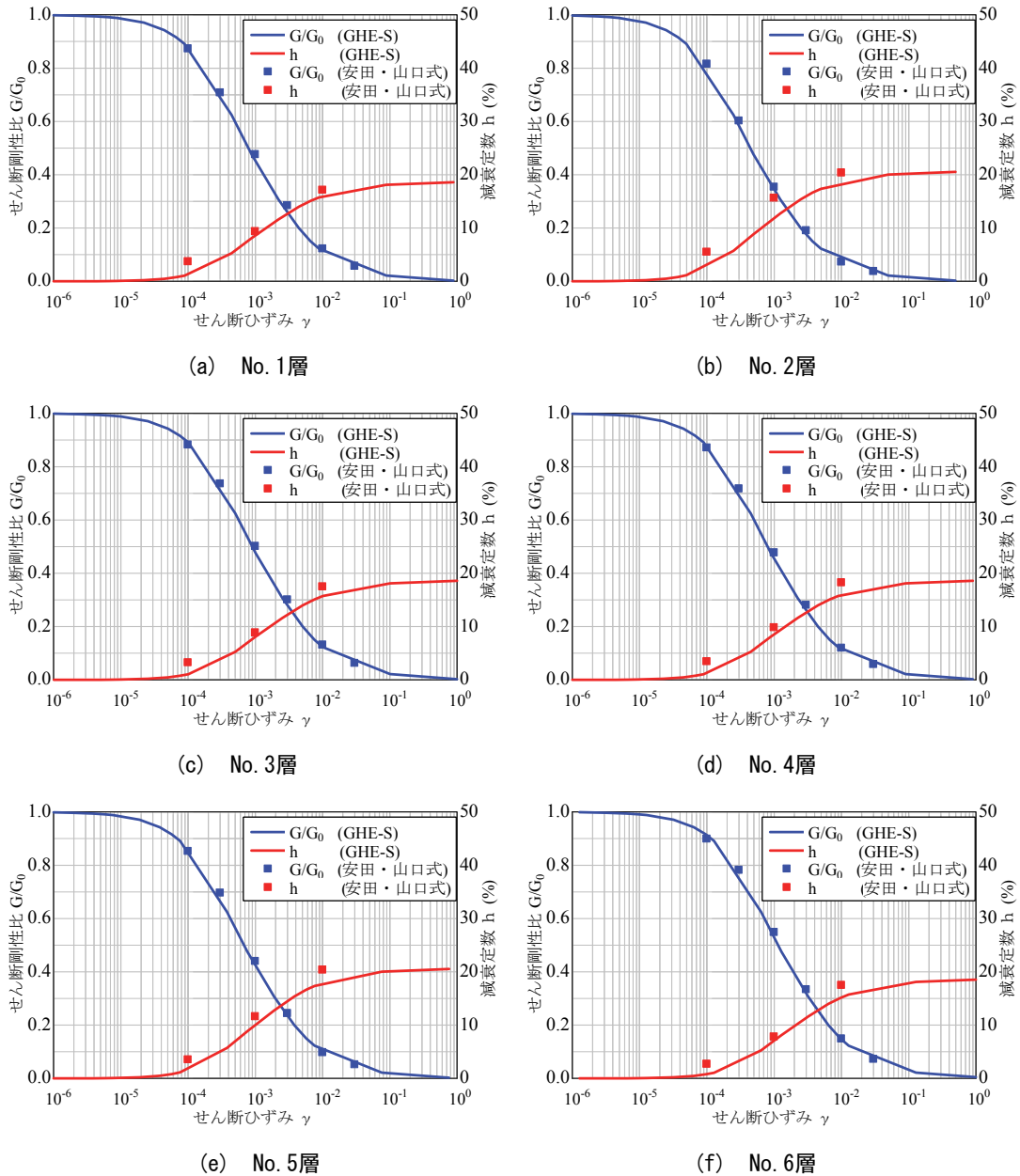
付図2-1 動的変形特性の設定結果（在来線地震計）その1
