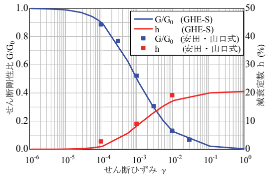
(f) No. 6層
