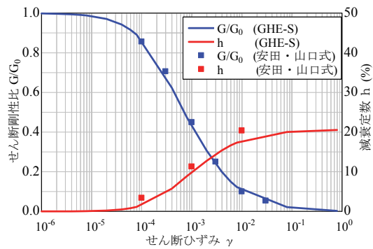
(d) No. 4層
