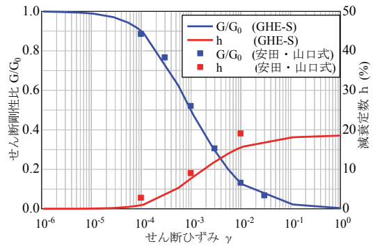
(d) No. 6層
