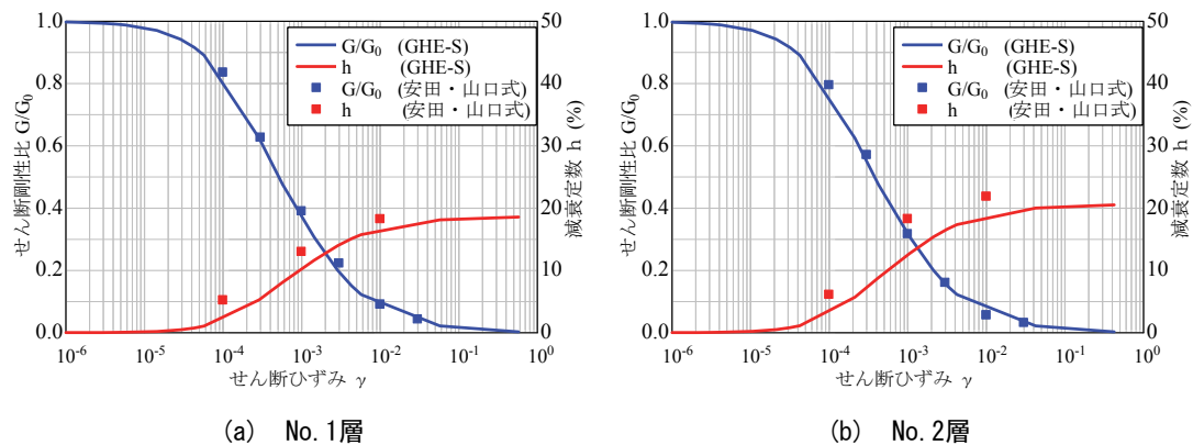
付図2-3 動的変形特性の設定結果（気象庁地震計）その1
