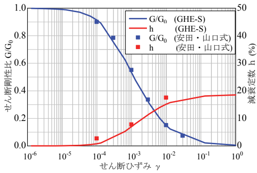
(e) No. 5層
