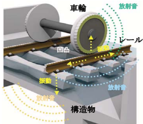
図3 転動音・構造物音予測手法
