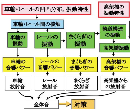
図3 転動音・構造物音予測手法
