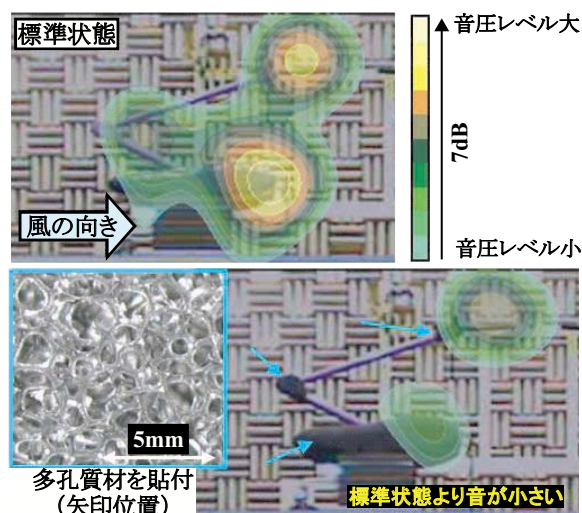
図2 多孔質材によるパンタグラフの空力音低減
