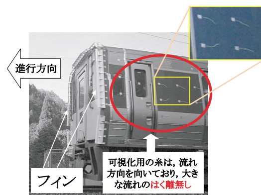
図4 在来線先頭車両の空気抵抗低減に関する試験
