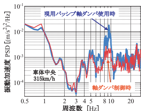
図3 軸ダンパの制御による車体上下振動低減効果
