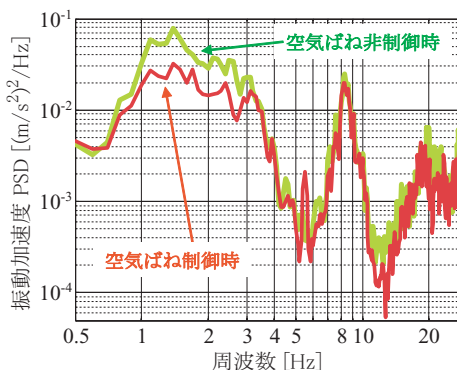
図6 空気ばねの減衰制御による車体上下振動低減効果
