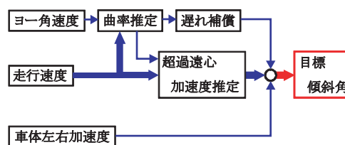
図9 制御ブロック線図
