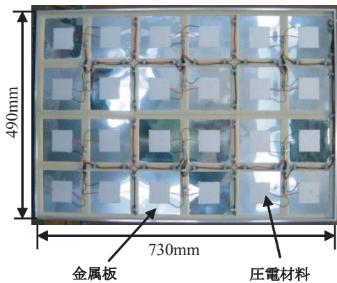
図11 騒音低減パネル
