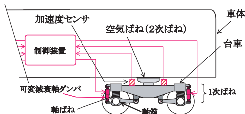
図1 可変減衰軸ダンパを用いた上下制振制御システム
