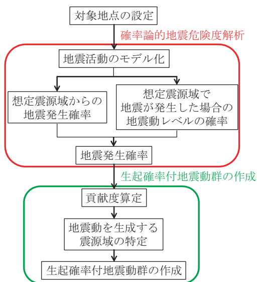
図1 本手法の概略的な流れ
