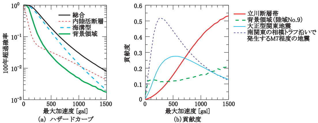
図5 対象地点における地震危険度解析結果
