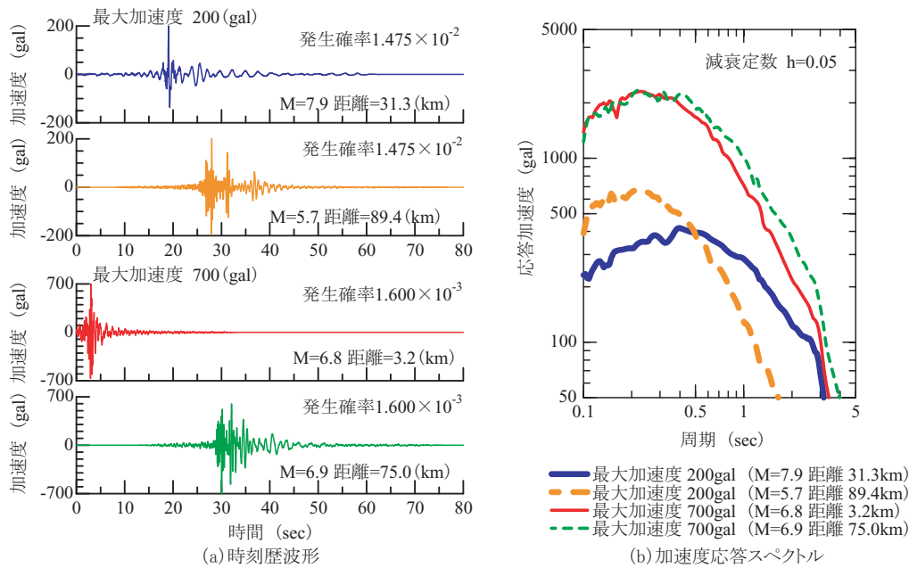
図6 生起確率付地震動群の例
