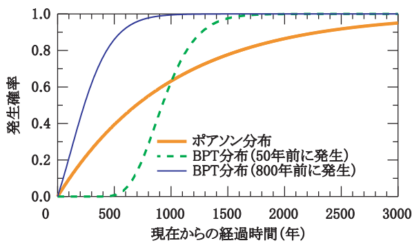
図3 地震発生確率の試算例 ( \mu=1000, \alpha=0.24 )
