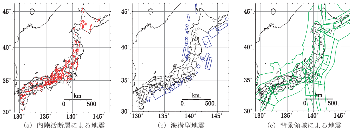
図2 地震活動のモデル化
