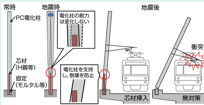
芯材を挿入する倒壊防止工法の概要
